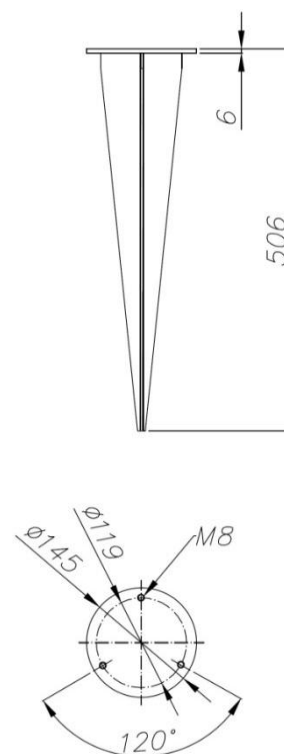
Fixation en sol naturel
