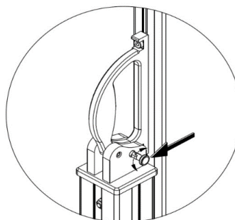
Alignement de la partie inférieure de la barre avant/frontale sur l'aimant dans le montant
