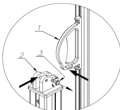
Blocage de la poignée dans le support de poignée
